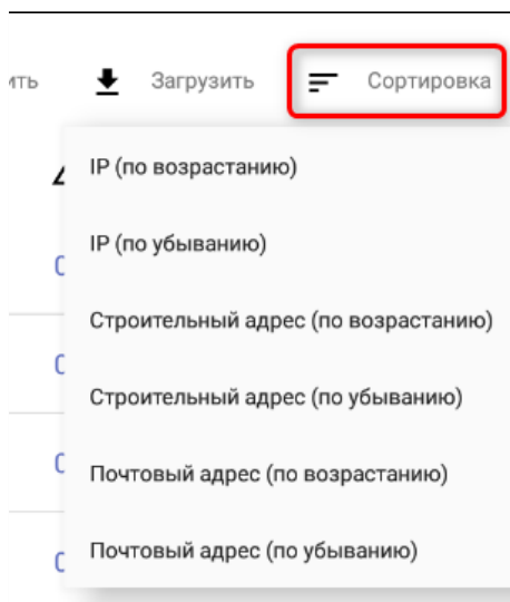
Рисунок 12 - Варианты сортировки
