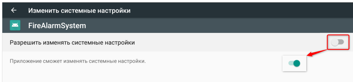
Рисунок 6 - Установка разрешения
