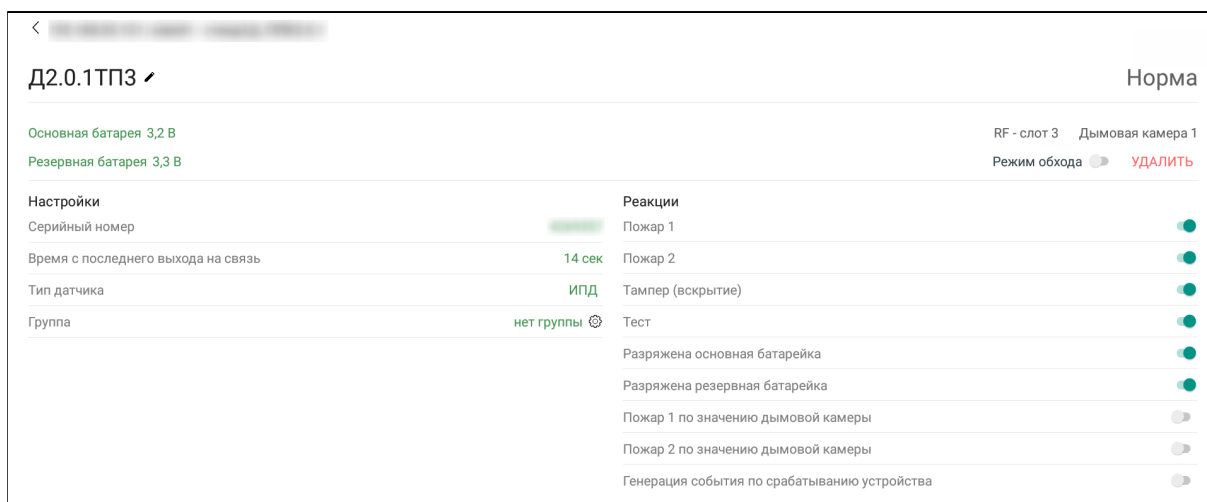
Рисунок 33 - Настройки RF-устройства
