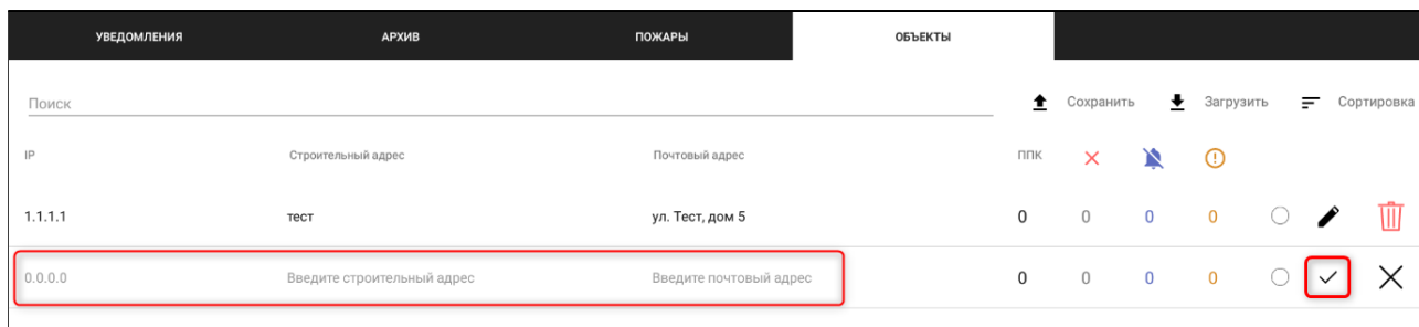
Рисунок 11 - Добавление объекта
