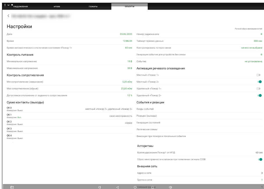
Рисунок 24 - Настройки ППК
