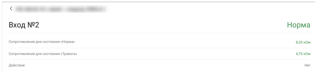
Рисунок 26 - Настройки Входа
