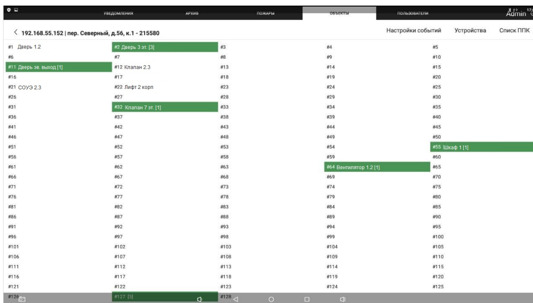
Рисунок 13 - Страница События
