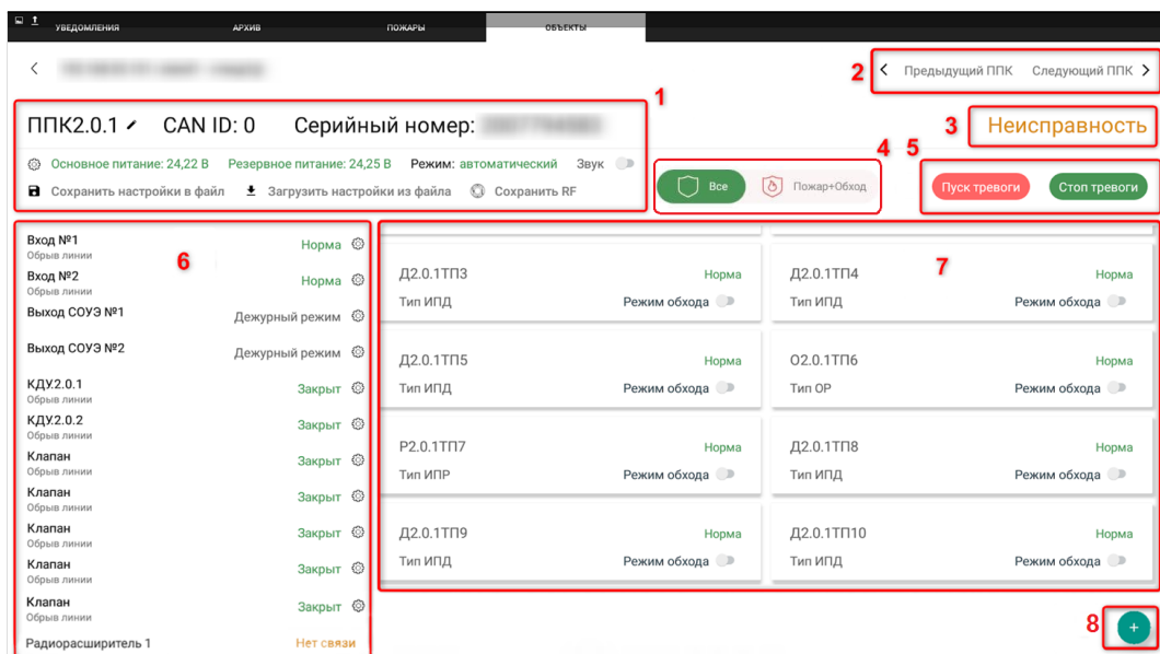
Рисунок 22 - Окно ППК
