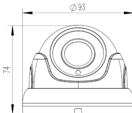
Рис. 2 – Габаритные размеры видеокамеры
