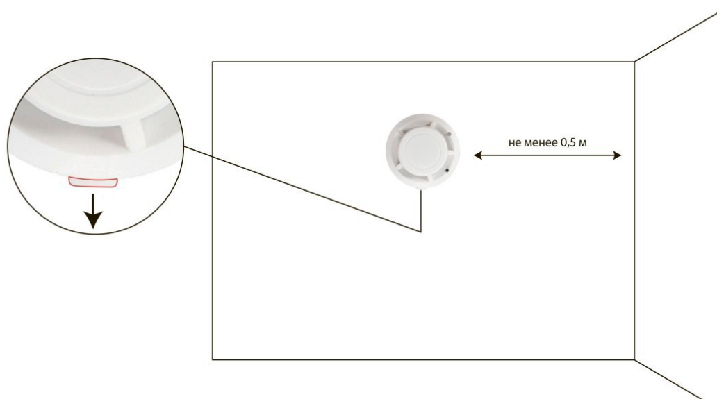
Рисунок 5 - Размещение извещателя на вертикальной поверхности
