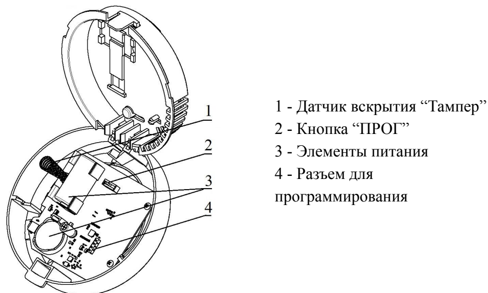
Рисунок 2 - Внутреннее устройство извещателя
